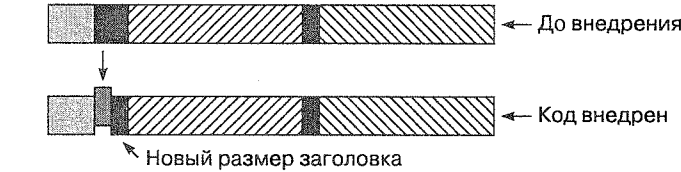
Рис. 4.7. Внедрение информации в свободное пространство хвоста РЕ-заголовка
