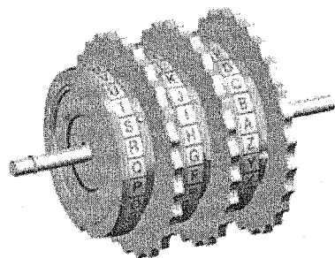
Рис. 1.13. Три последовательно соединенных ротора
