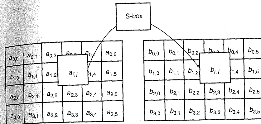
Рис. 1.22. ByteSub действует на каждый байт состояния
