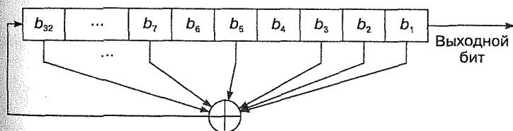
Рис. 3.11. 32-битовый РгСсЛОС с максимальной длиной
