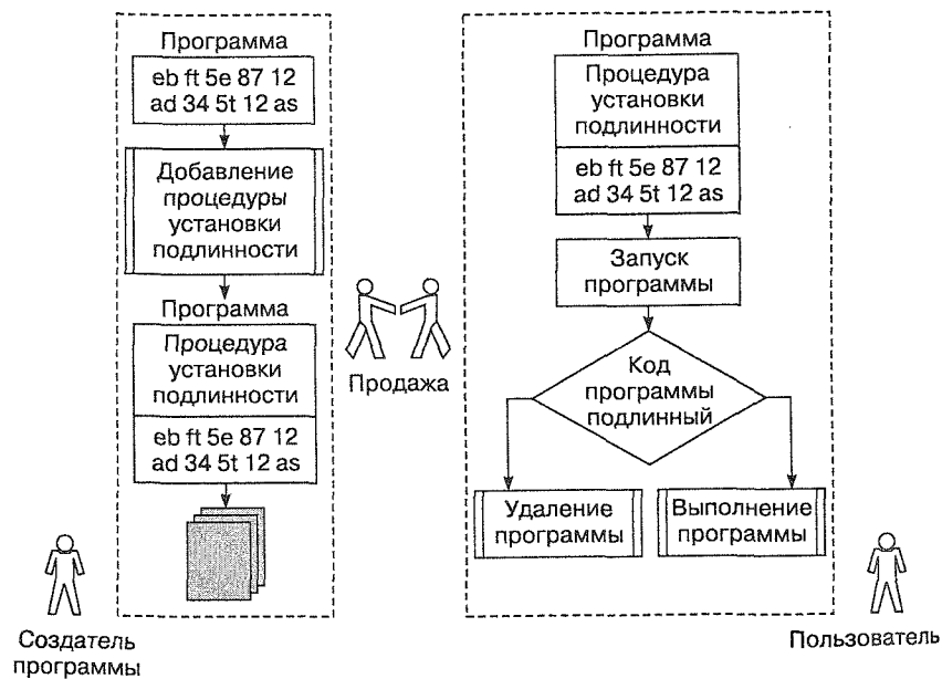
Рис. 4.2. Установка подлинности кода
