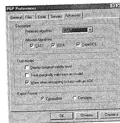
Рис. 2.8. Окно PGP Preferences
