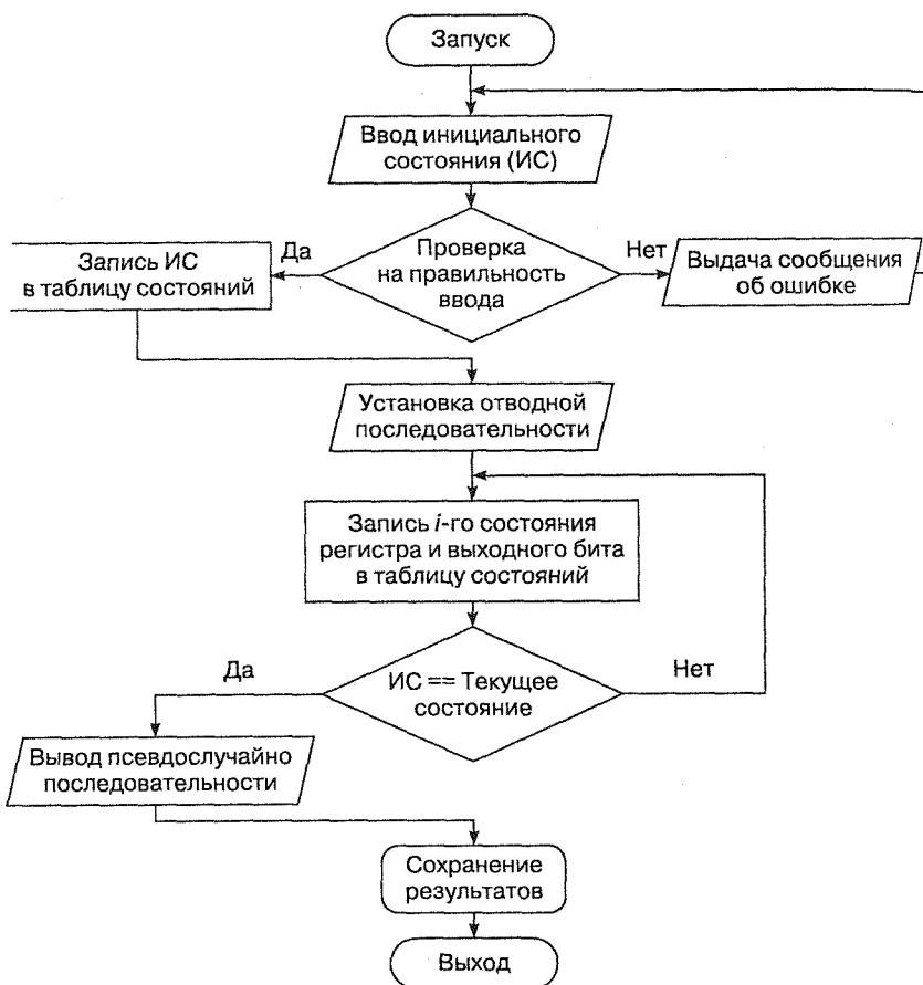
Рис. 3.12. Обобщенная схема алгоритма РгСсЛОС
