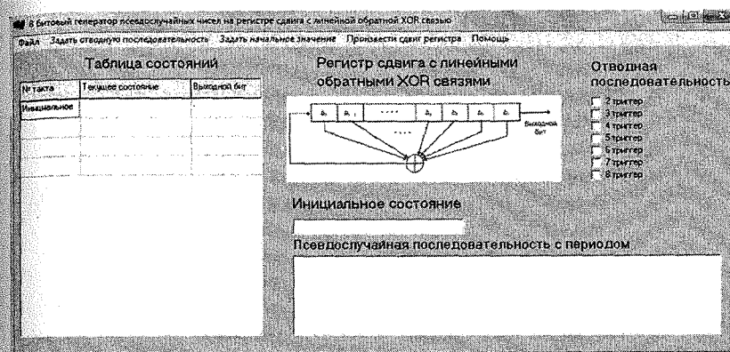
Рис. 3.13. Главное окно программы
