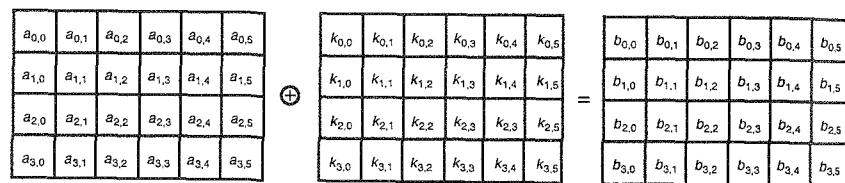
Рис. 1.24. Операция добавления циклового ключа
