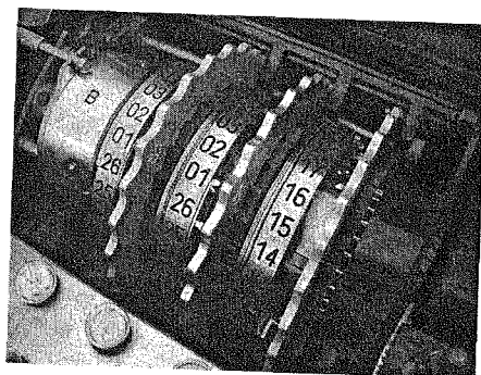
Рис. 1.14. Роторы энигмы в собранном состоянии. Три подвижных ротора помещены между двумя неподвижными деталями: входное кольцо и рефлексор (помечен «В» слева)
