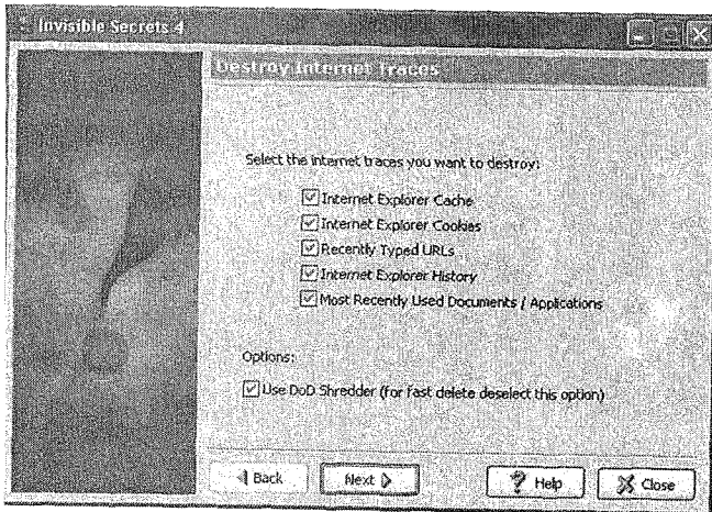
Рис. 4.47. Уничтожение ссылок
