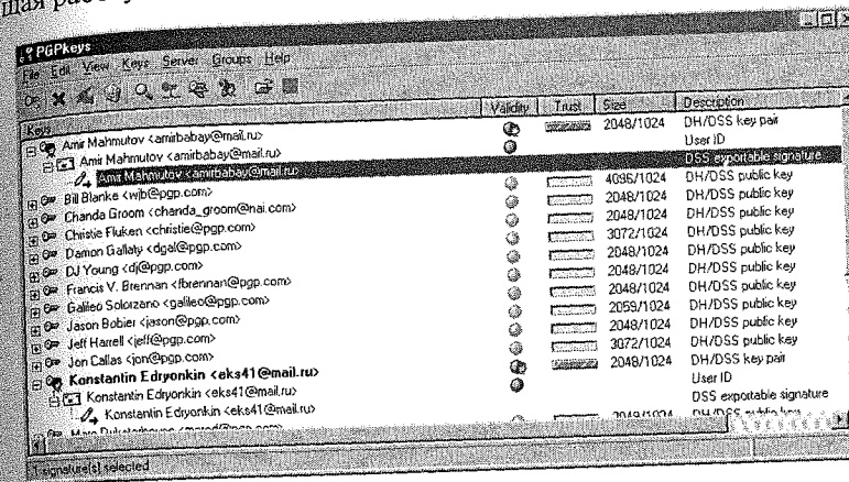
Рис. 2.7. Окно PGPkeys
