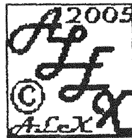
Рис. 4.22. Внедряемый ЦВЗ
