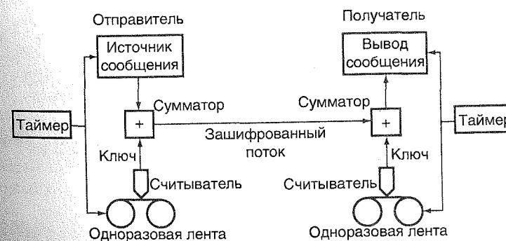
Рис. 1.1. Схема шифрования методом Вернама
