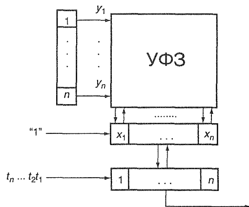
Рис. 2.5. Схема реализации шифрующего автомата скользящей перестановки
