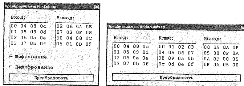
Рис. 1.28. Окна преобразований MixColumn и AddRoundKey
