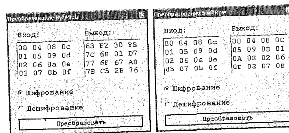
Рис. 1.27. Окна преобразований ByteSub и ShiftRow
