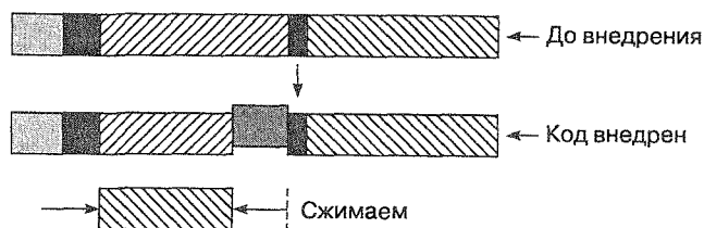
Рис. 4.13. Внедрение кода путем сжатия секции
