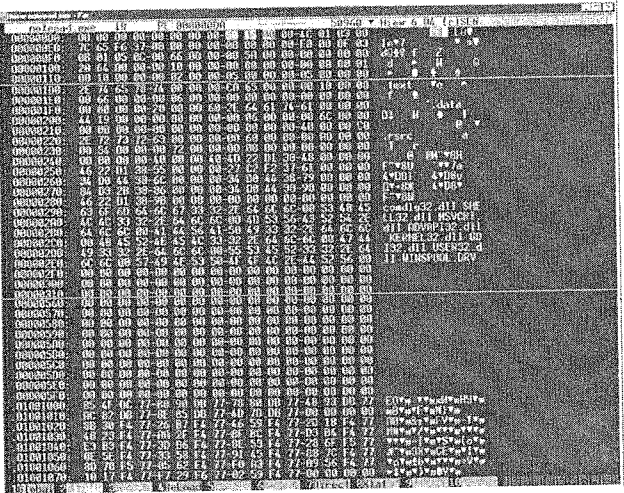
Рис. 4.8. Типичный РЕ-заголовок файла
