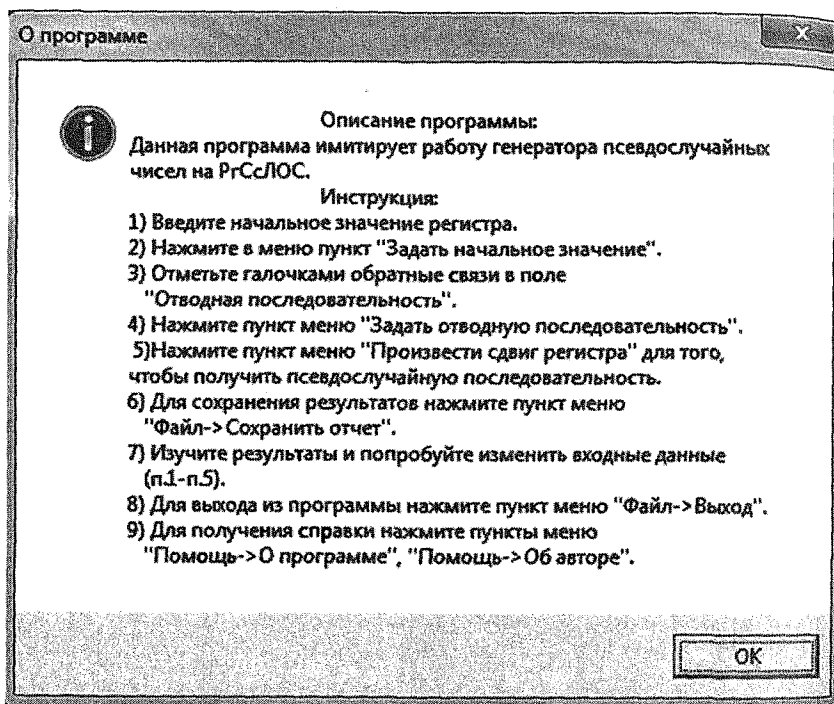
Рис. 3.21. О программе
