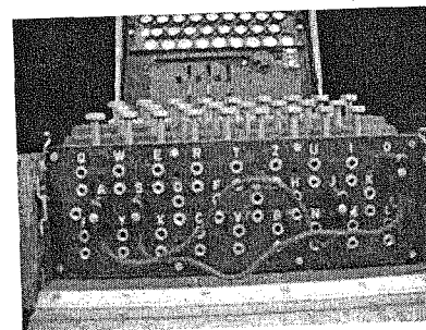
Рис. 1.15. Коммутационная панель «Энигмы»
